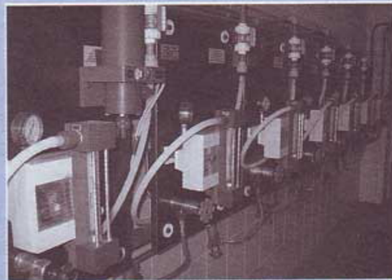
Хлораторы AXV-1000 производства ФСП "КРАВТ" на водозаборе МУП "Водоканал", г. Волжский
